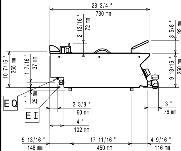
Oldalnézet
